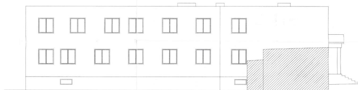
Elewacja północno-zachodnia
